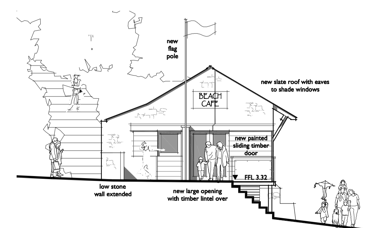
SW Elevation
