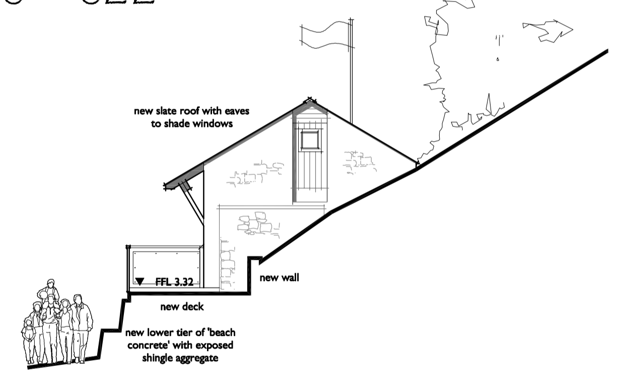
NE Elevation
